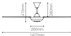
RCF-FORZA56-5BL 56"
