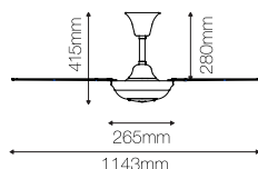
RCF-FORZA45-5BL 45"
